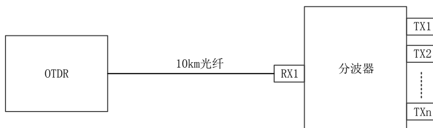
图16 光反射系数测量框图
