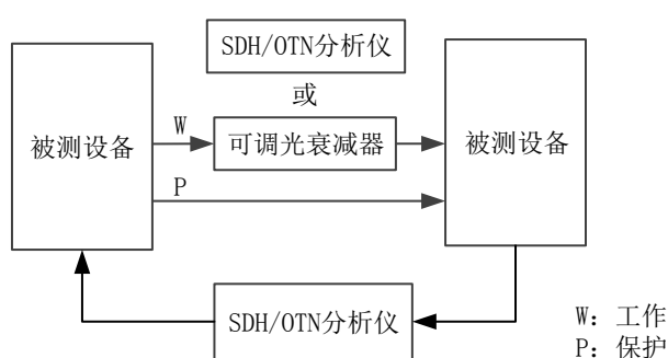
图22 保护倒换测量框图
