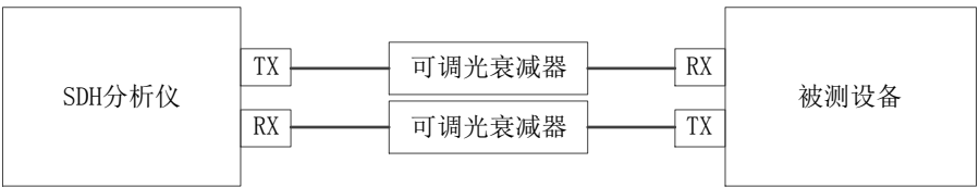
图10 输出抖动测量框图
