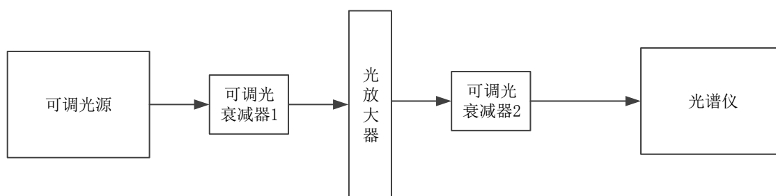
图17 增益测量框图
