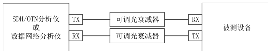
图21 误码/丢包性能测量框图
