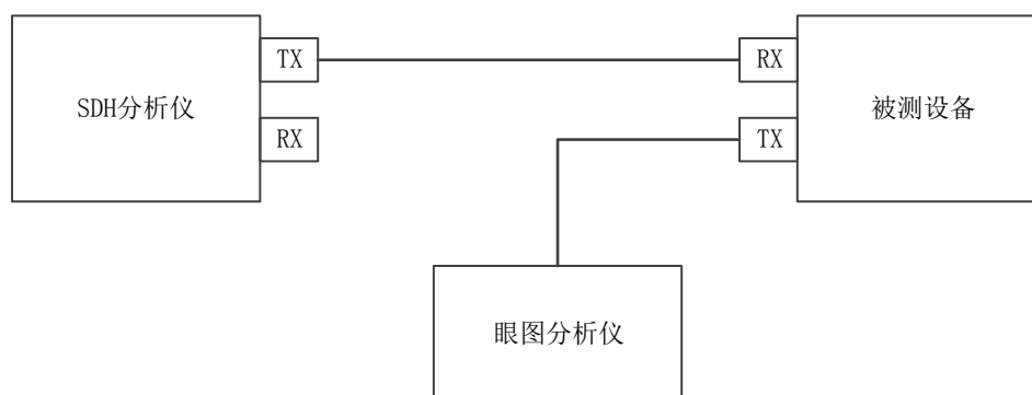
图8 眼图、最小消光比测量框图
