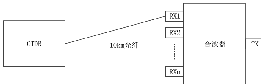
图13 光反射系数测量框图
