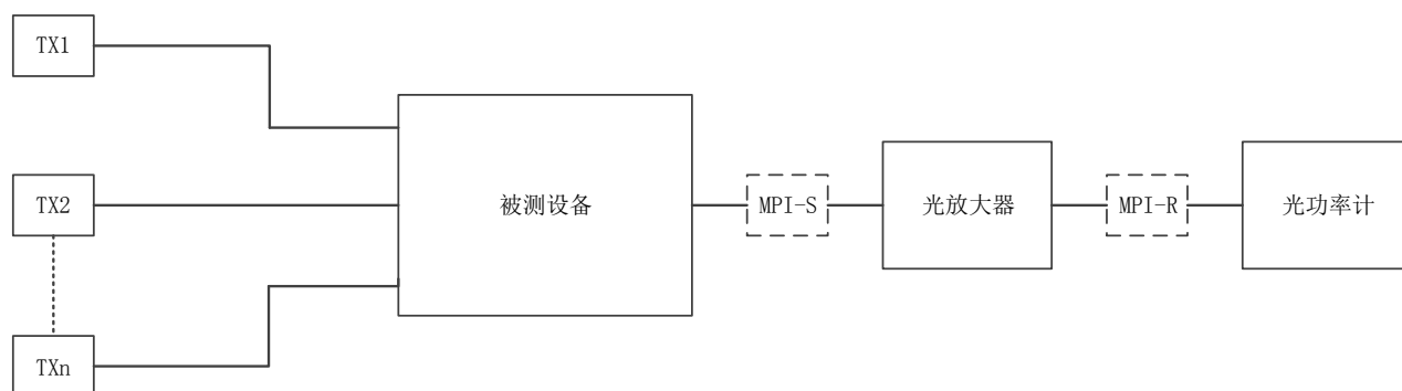
图4 总接收功率测量框图
