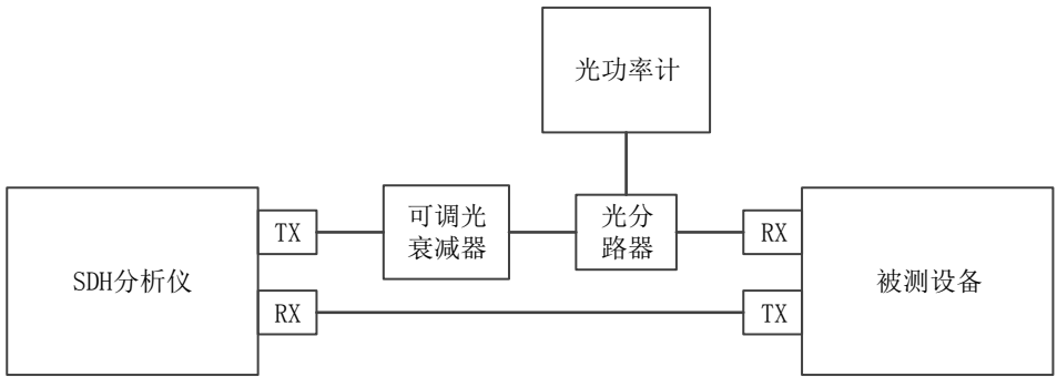
图9 接收机最差灵敏度、最大过载测量框图
