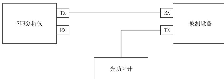
图7 平均发送光功率测量框图
