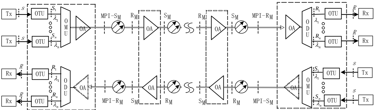
图1 WDM 系统功能模型框图
