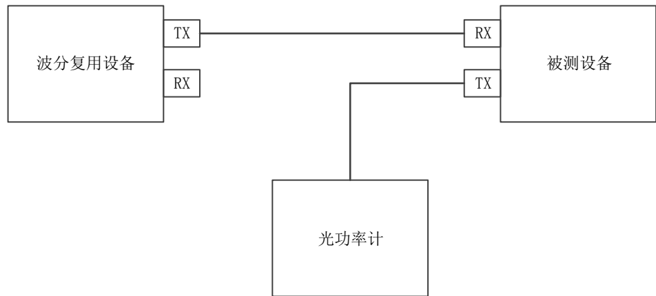
图19 信号发送光功率测量框图
