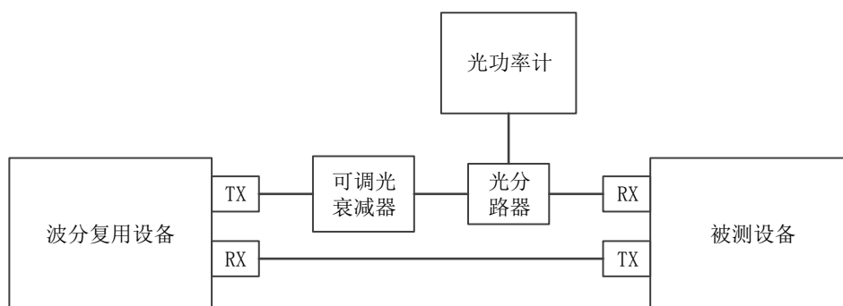
图20 最小接收灵敏度测量框图
