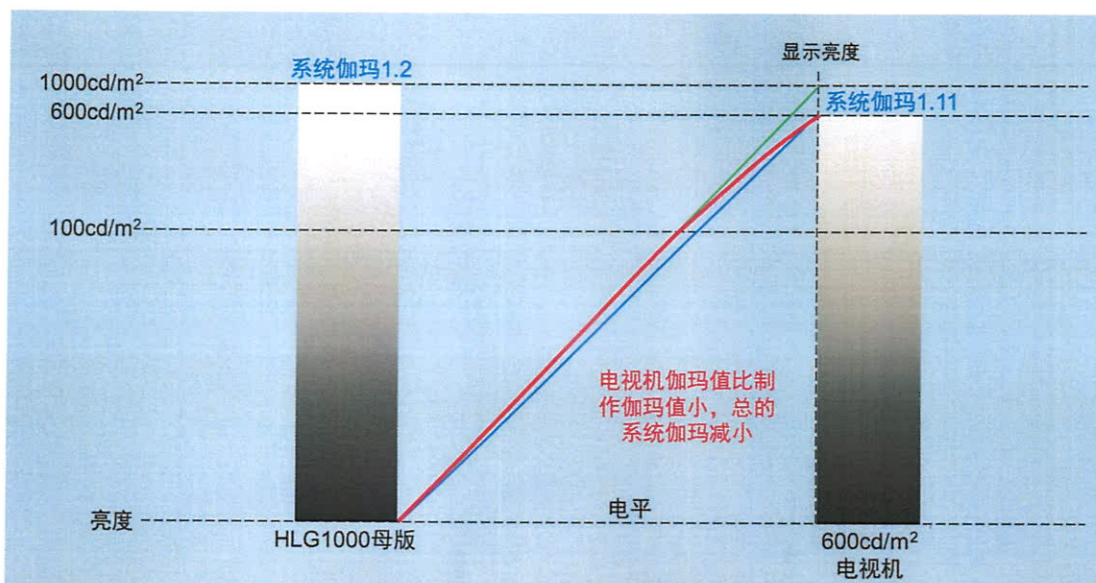
图 C.2 HLG 电视机亮度低于母版亮度
