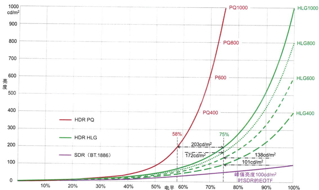
图 B.2 不同峰值亮度时 SDR 与 HDR 的 EOTF 特性
