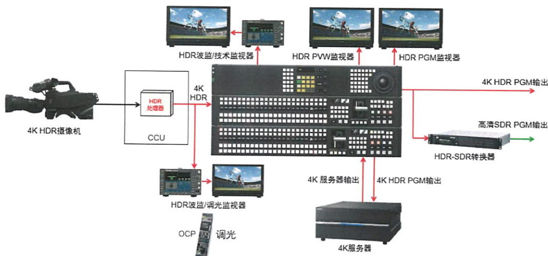
图4 4K HDR 制作系统：用 HDR 调光制作 HDR
