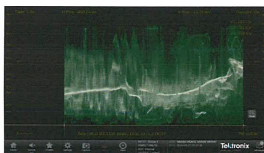
（b）测试序列 1 复合信号波形截图
